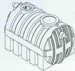
A1 MFR2-PE D(Ø) : 1200 H1 : 1200 L : 2060
