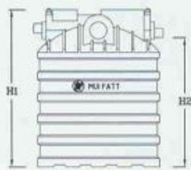
A2 MF6-PE D(Ø) : 1450 H1 : 1530
